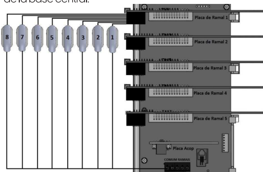
Figura 8- Puntos de Conexión de los internos PCD-40 y PCD-80
