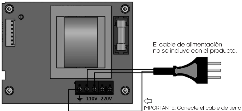
Figura 2- Esquema de la entrada de alimentación de 110 V IMPORTANTE: Conectar a tierra el punto de tierra de la fuente
